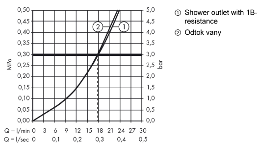
Průtokový diagram
