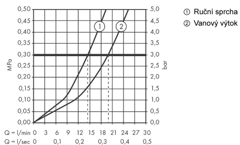
Průtokový diagram
