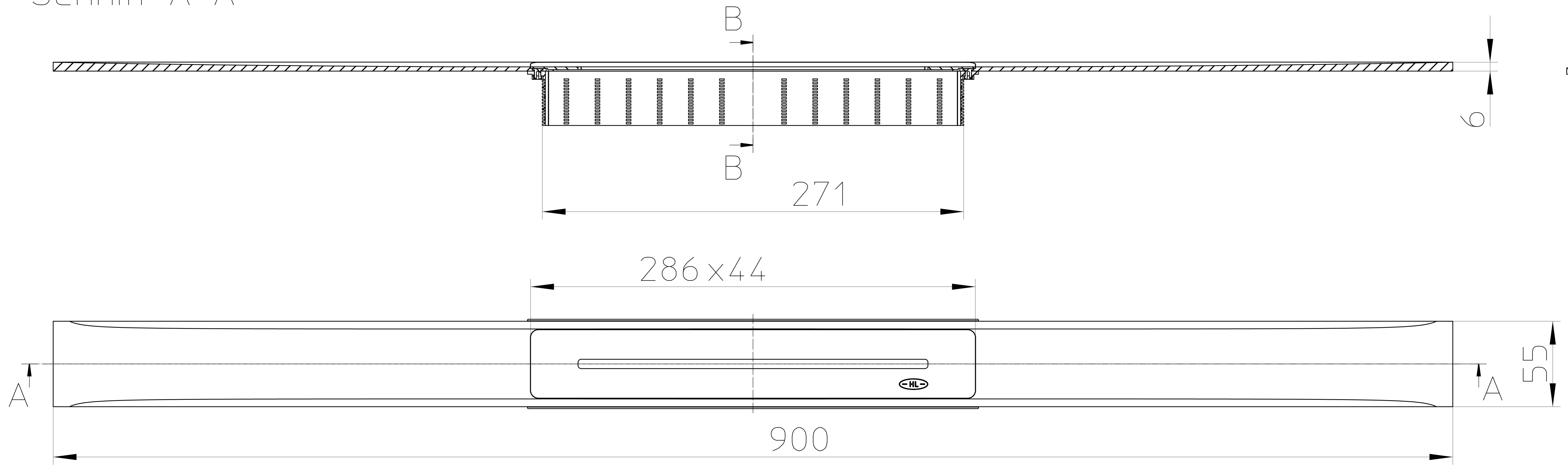
Schnitt A-A
