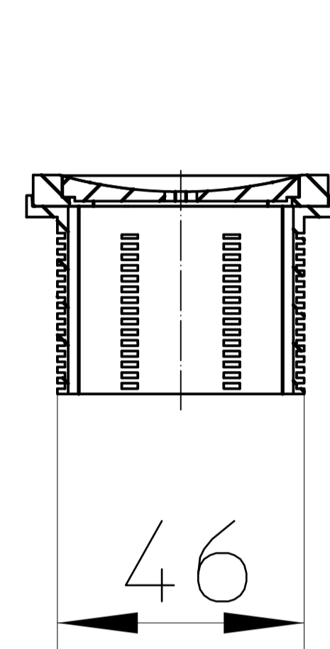
Schnitt B-B
