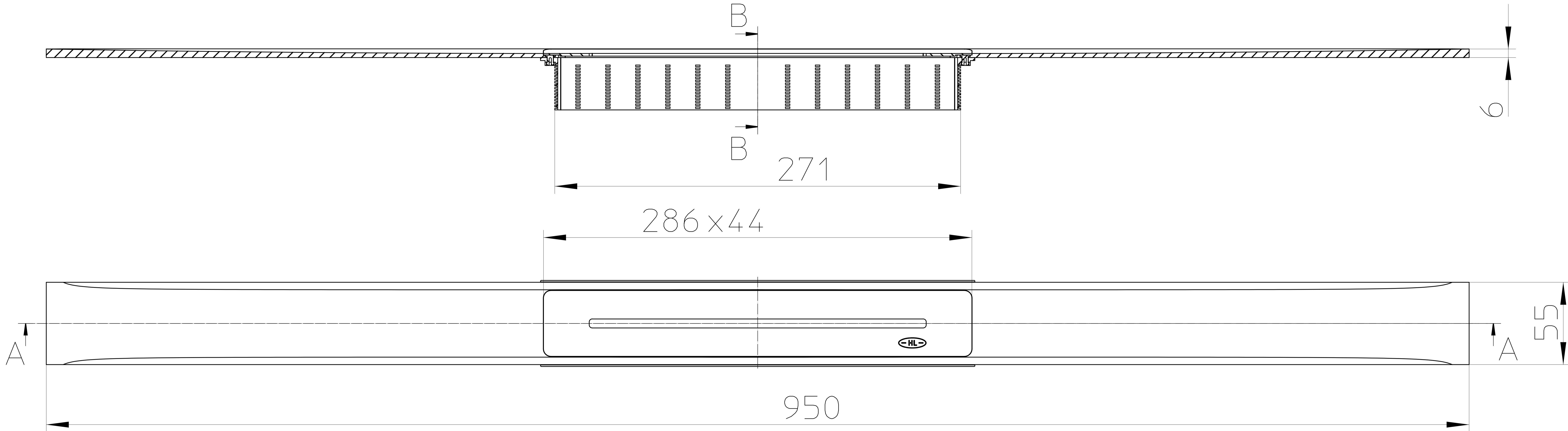
Schnitt A-A
