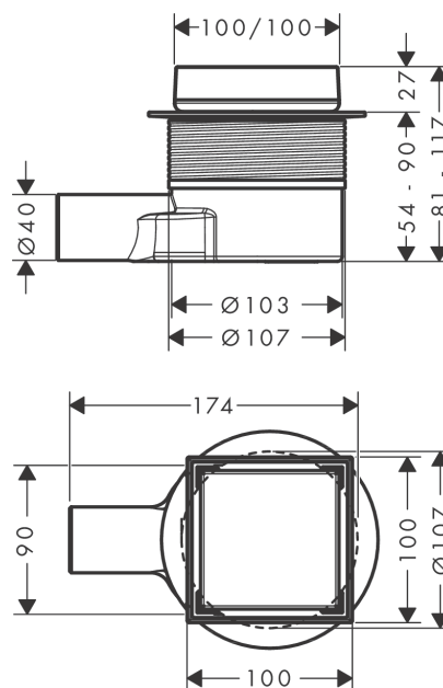
Kótovaný výkres
