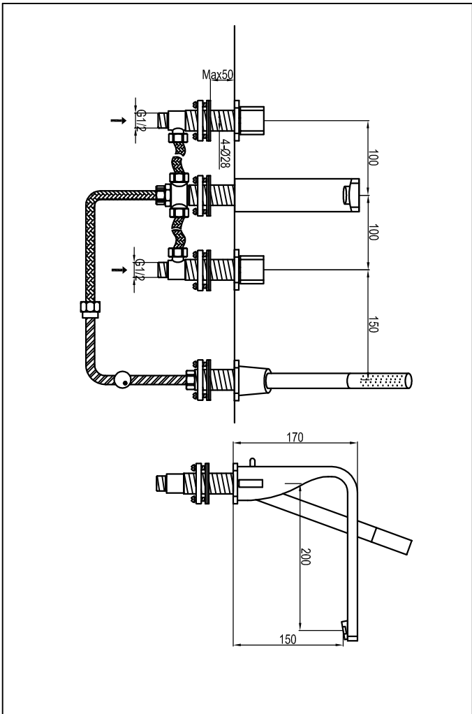
Technische Zeichnung
