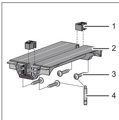
Obr. 7: spojovací kus, obsah dodávky
