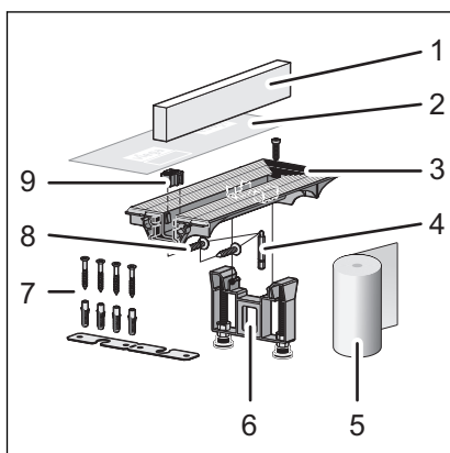
Obr. 8: uzavírací koncová tvarovka, obsah dodávky
