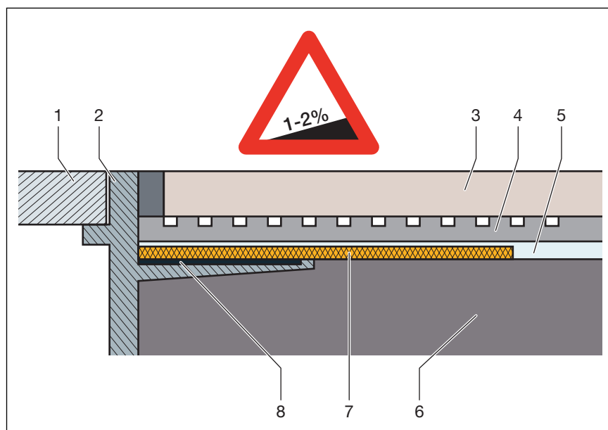
Obr. 11: schéma konstrukce spojené izolace – sklon potěru min. 1–2 %
