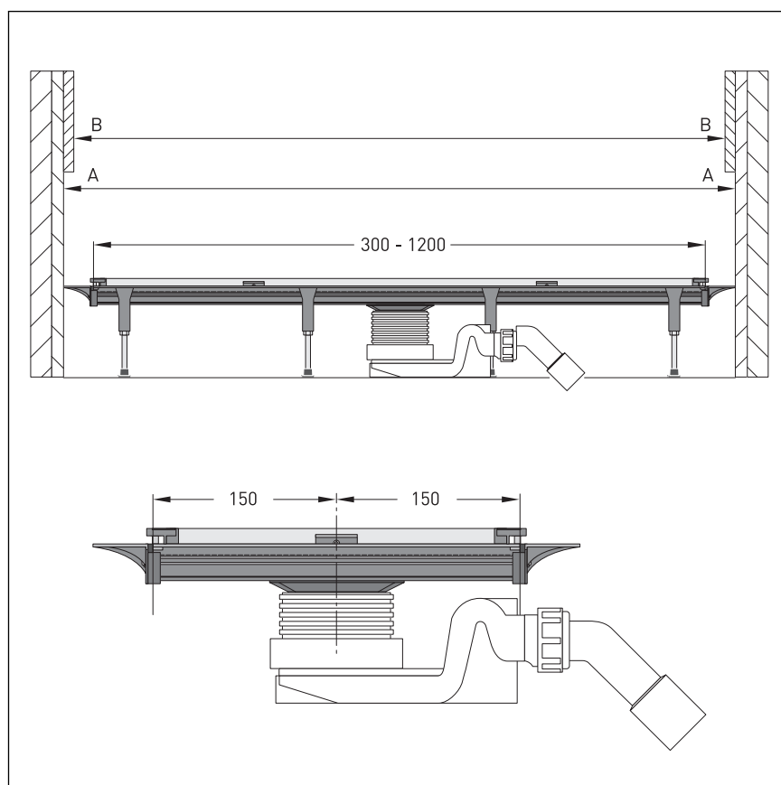
Obr. 18: rozměry výklenku
