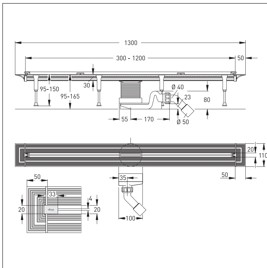
Obr. 14: rozměry základního tělesa základní model
