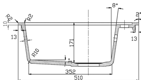
REZ B-B
