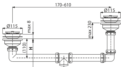
A454P: H=270-370
