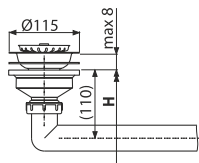
A453P: H=270-370
