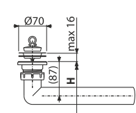
A449: H=220-325 A449P: H=265-325
