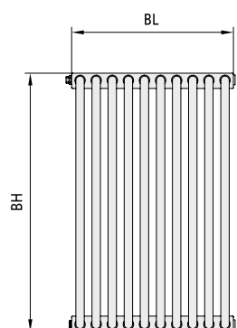
Čelní pohled
