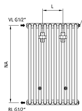
Pohled zezadu
