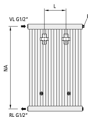
Pohled zezadu
