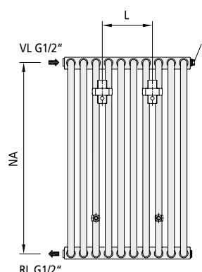
Pohled zezadu
