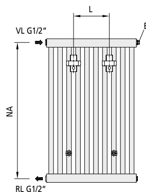
Pohled zezadu
