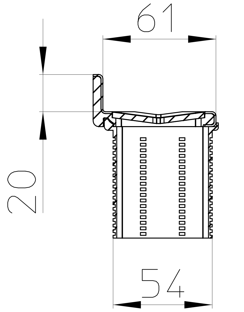
Schnitt B-B
